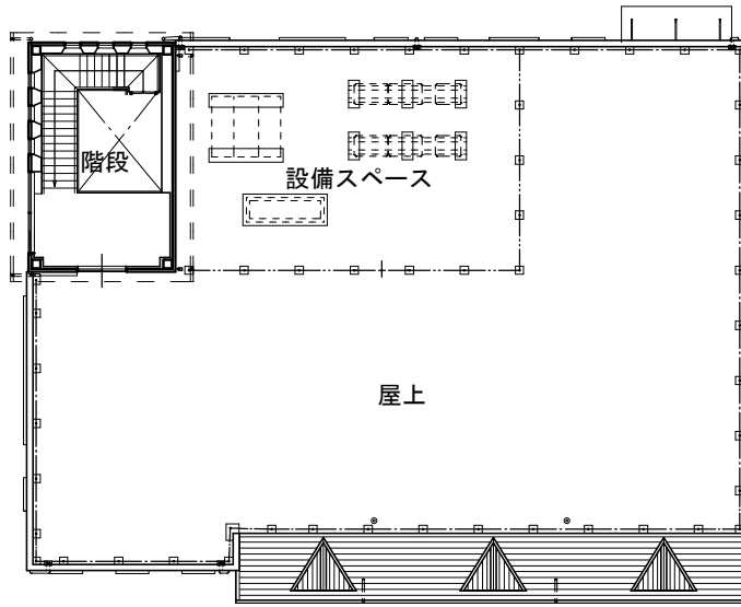
PH階平面図
