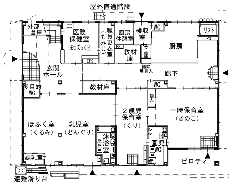
1階平面図
