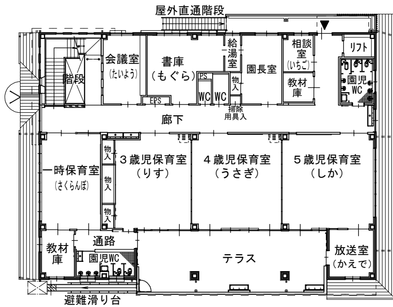
2階平面図
